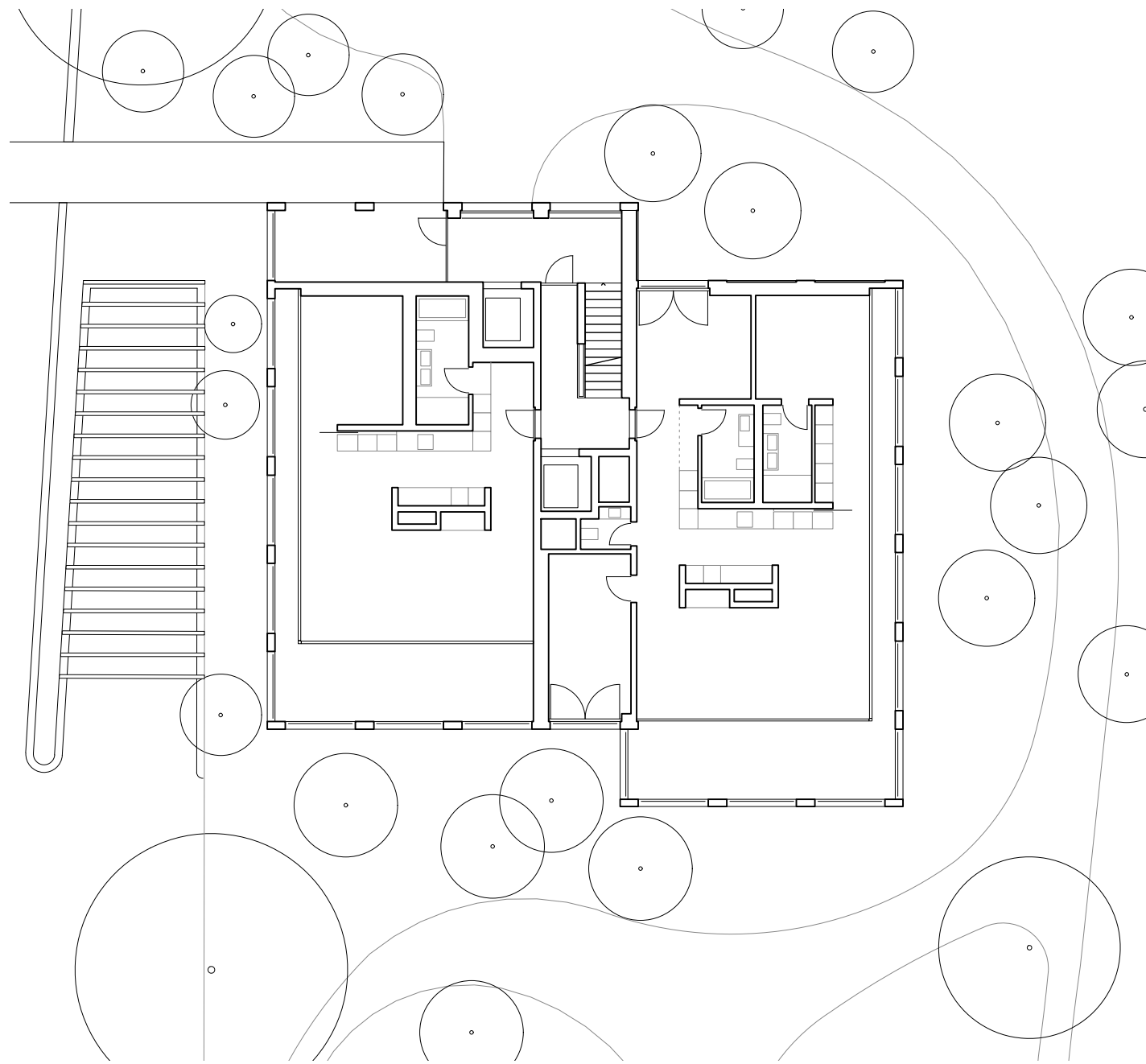
Erdgeschoss 1:200
