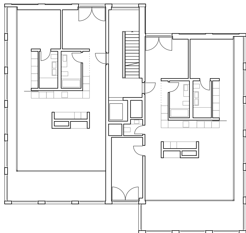
2.-3. Obergeschoss 1:200
