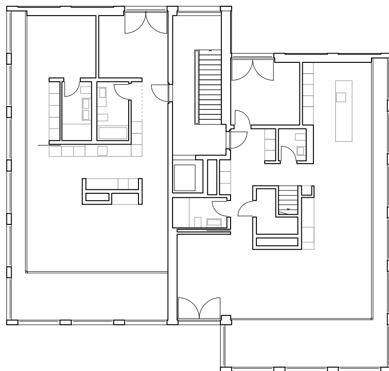
4. Obergeschoss 1:200
