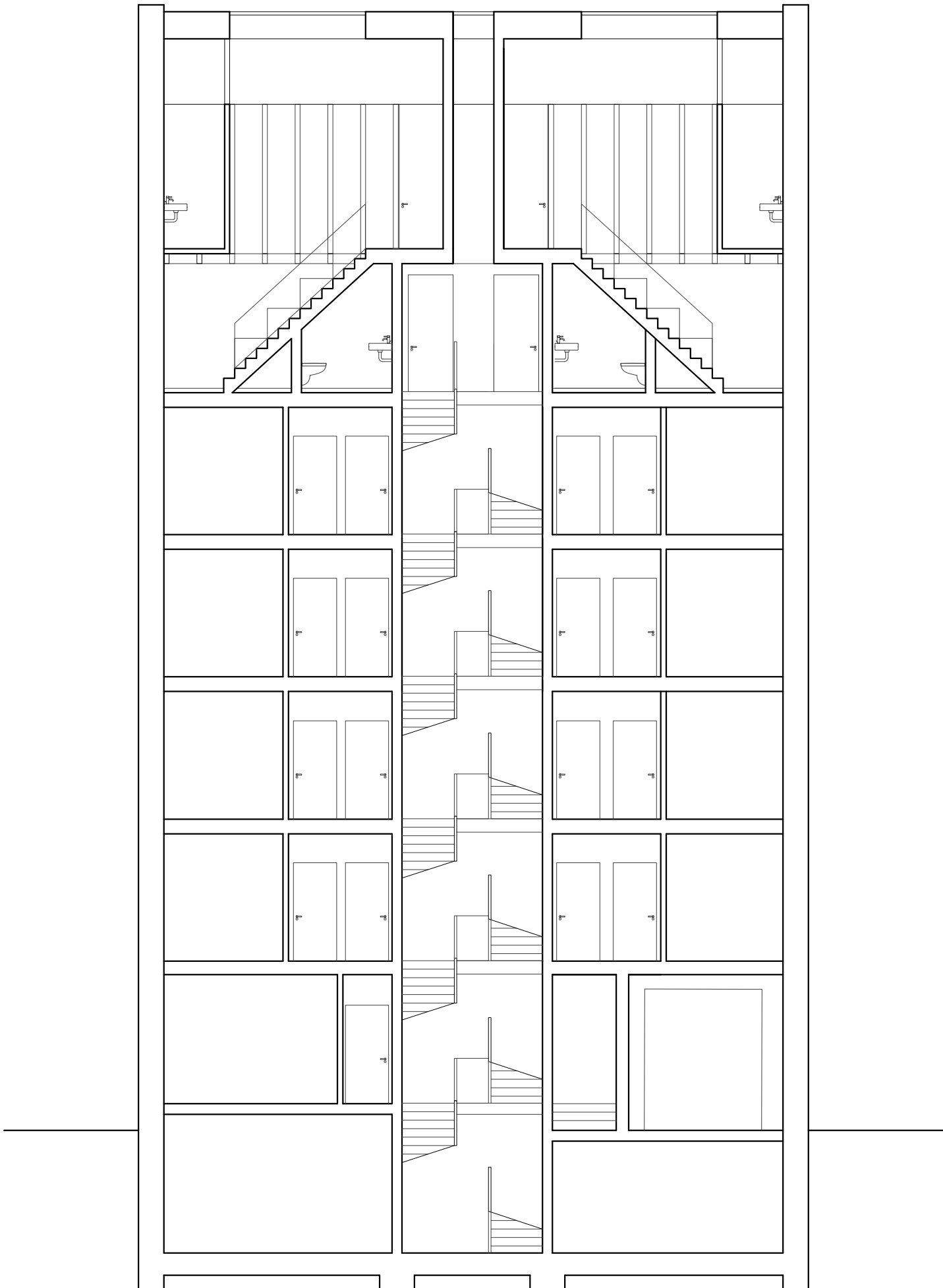
Längsschnitt
