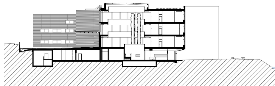
Querschnitt Eingang - Foyer
