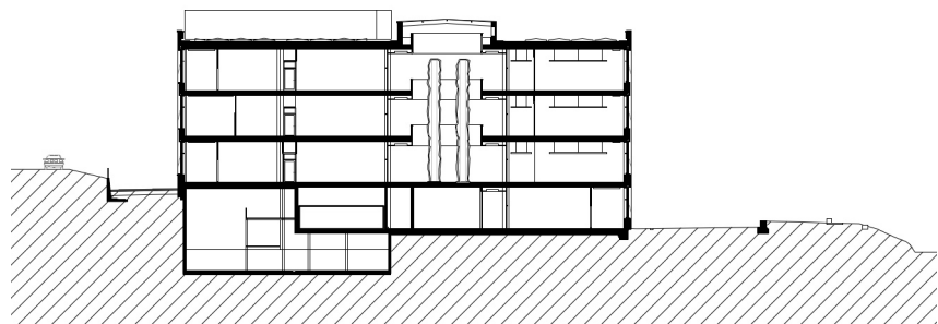
Querschnitt Büro - Labor
