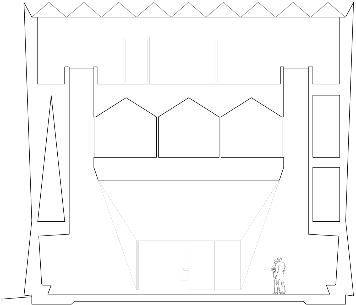
Coupe C-C
