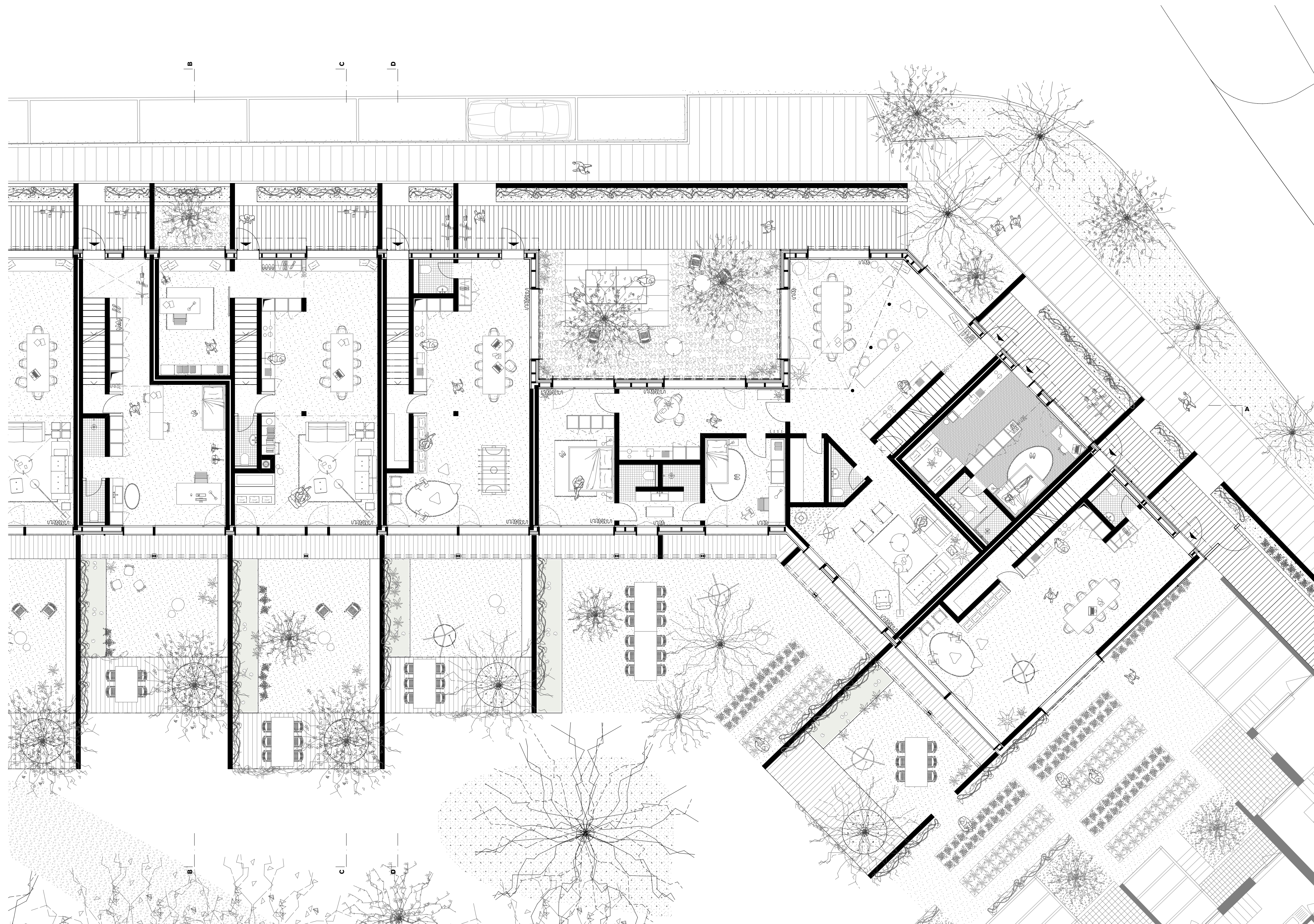
Raumtypologie Erdgeschoss 1:100
