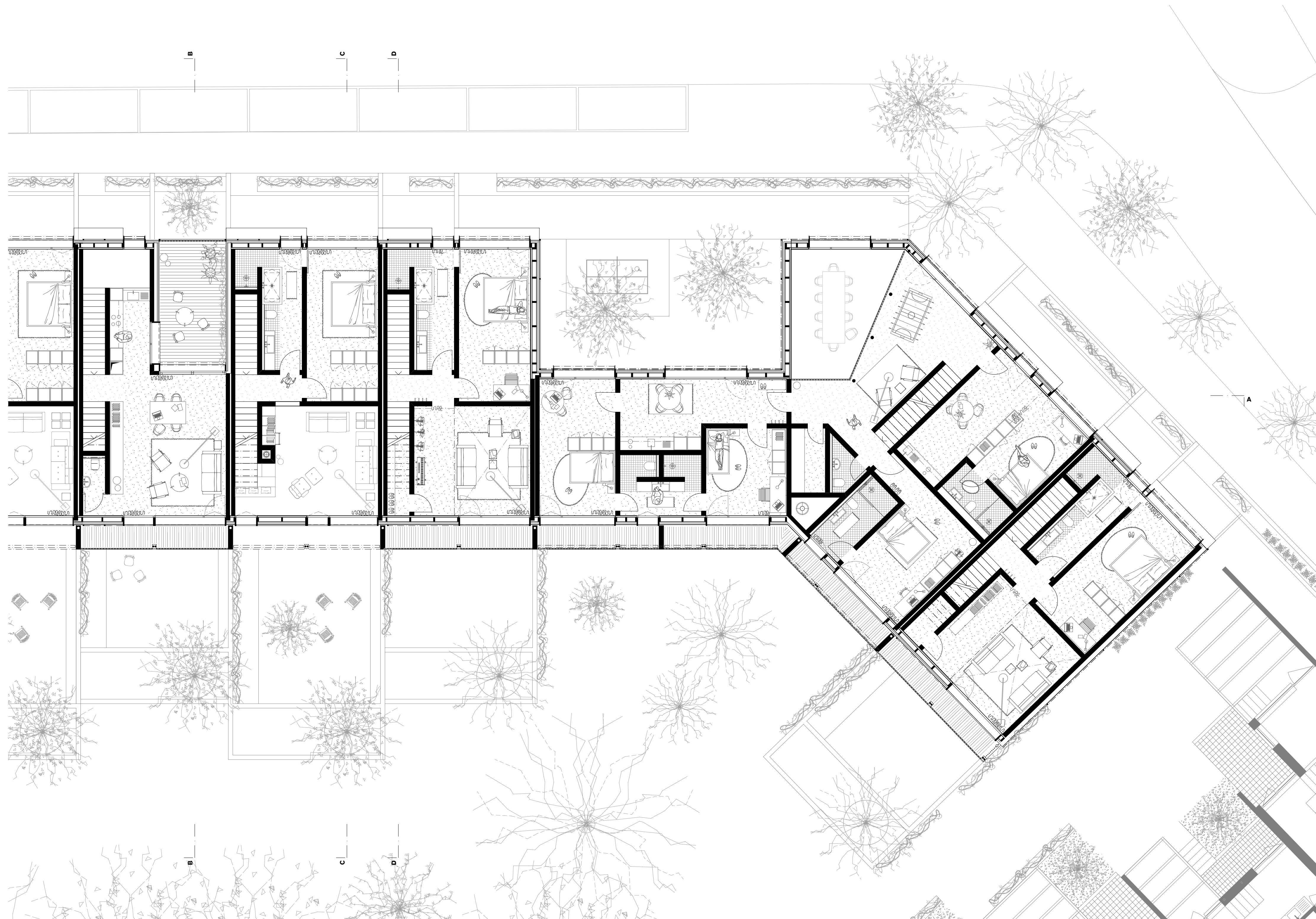
Raumtypologie 1. Obergeschoss 1:100
