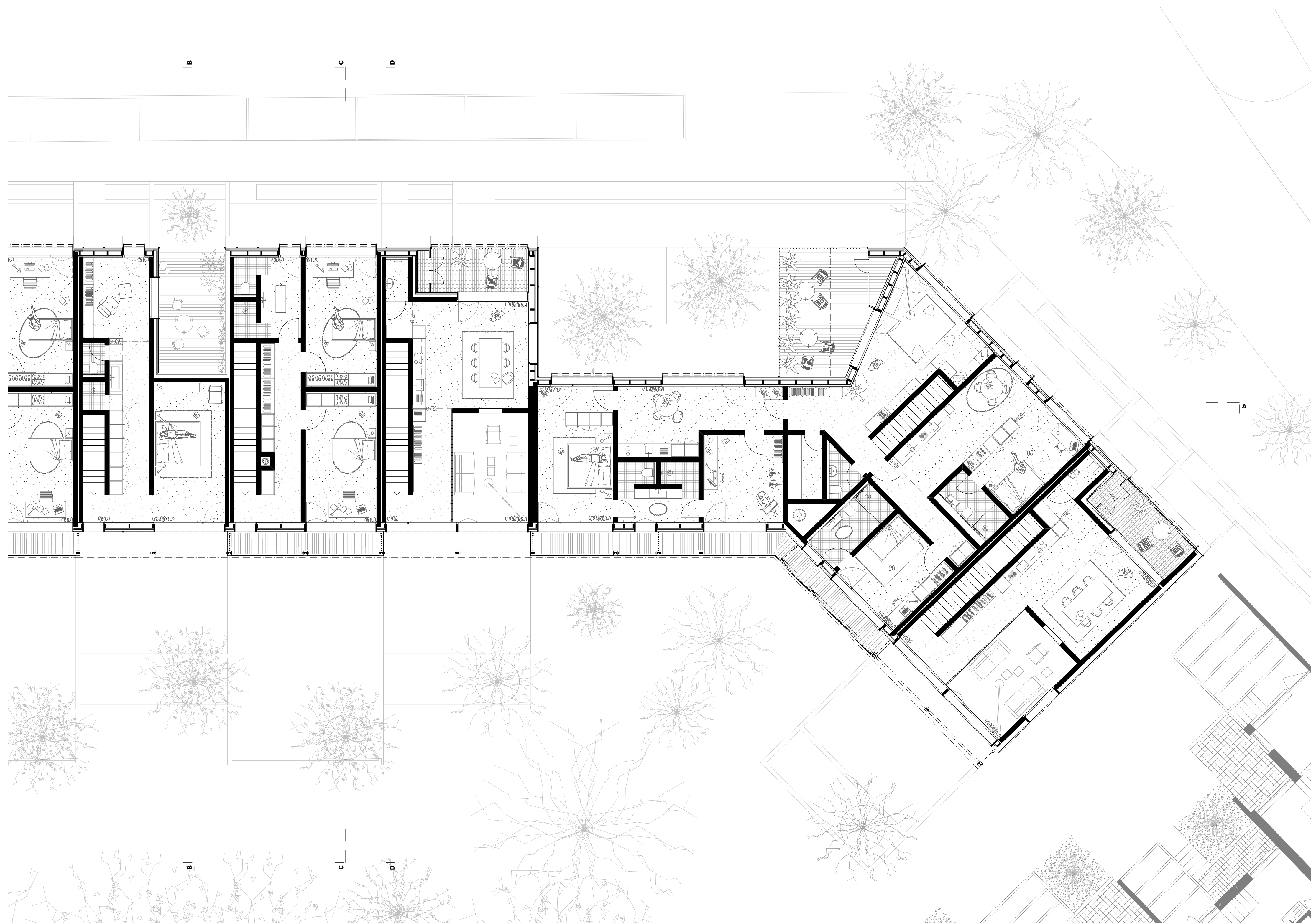
Raumtypologie 2. Obergeschoss 1:100
