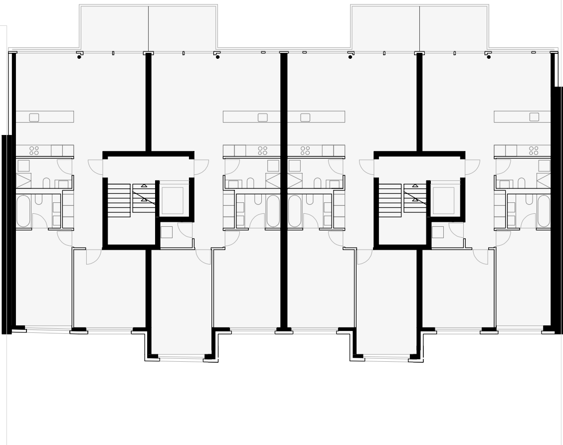
Grundriss 1. Obergeschoss
