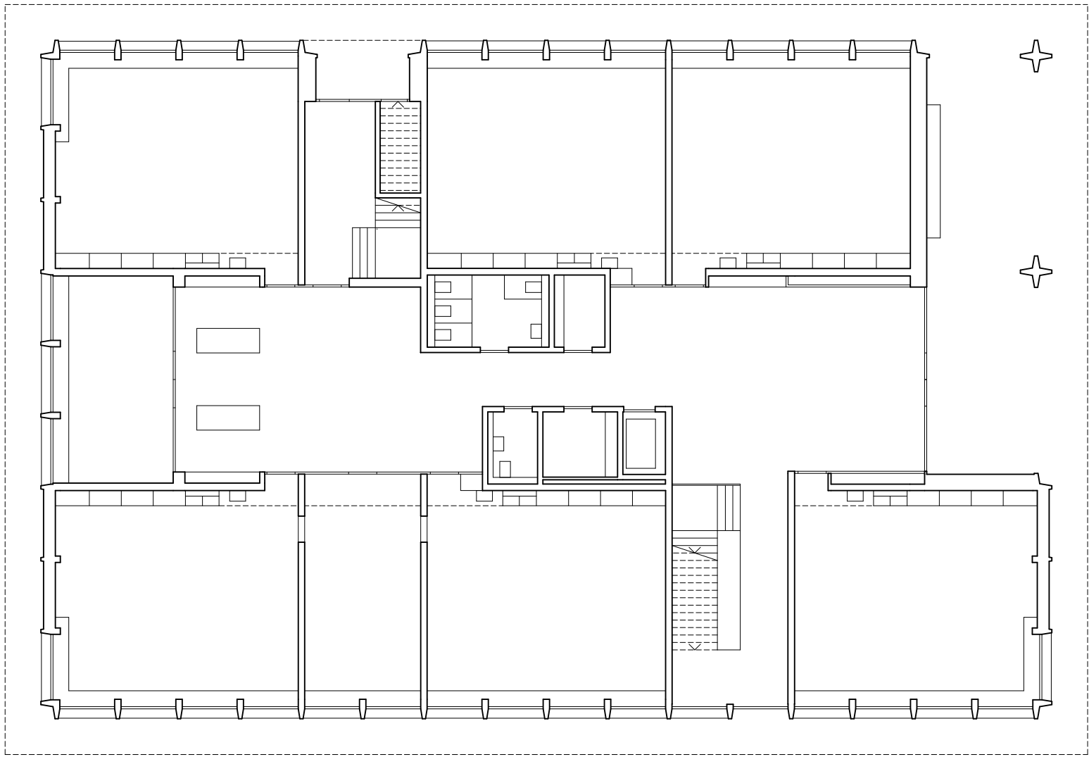
Erdgeschoss 1:200
