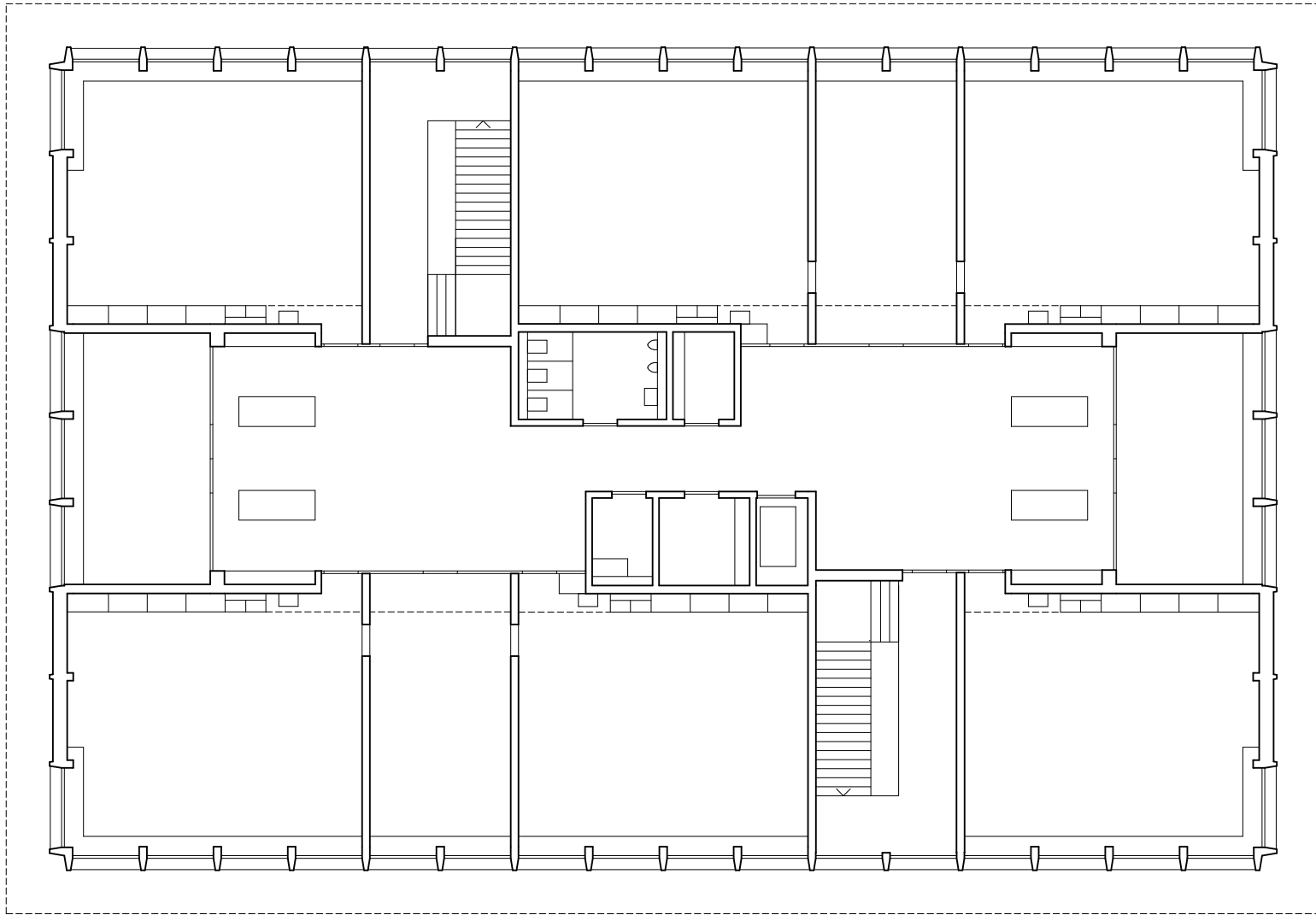
Obergeschoss 1:200 ↻
