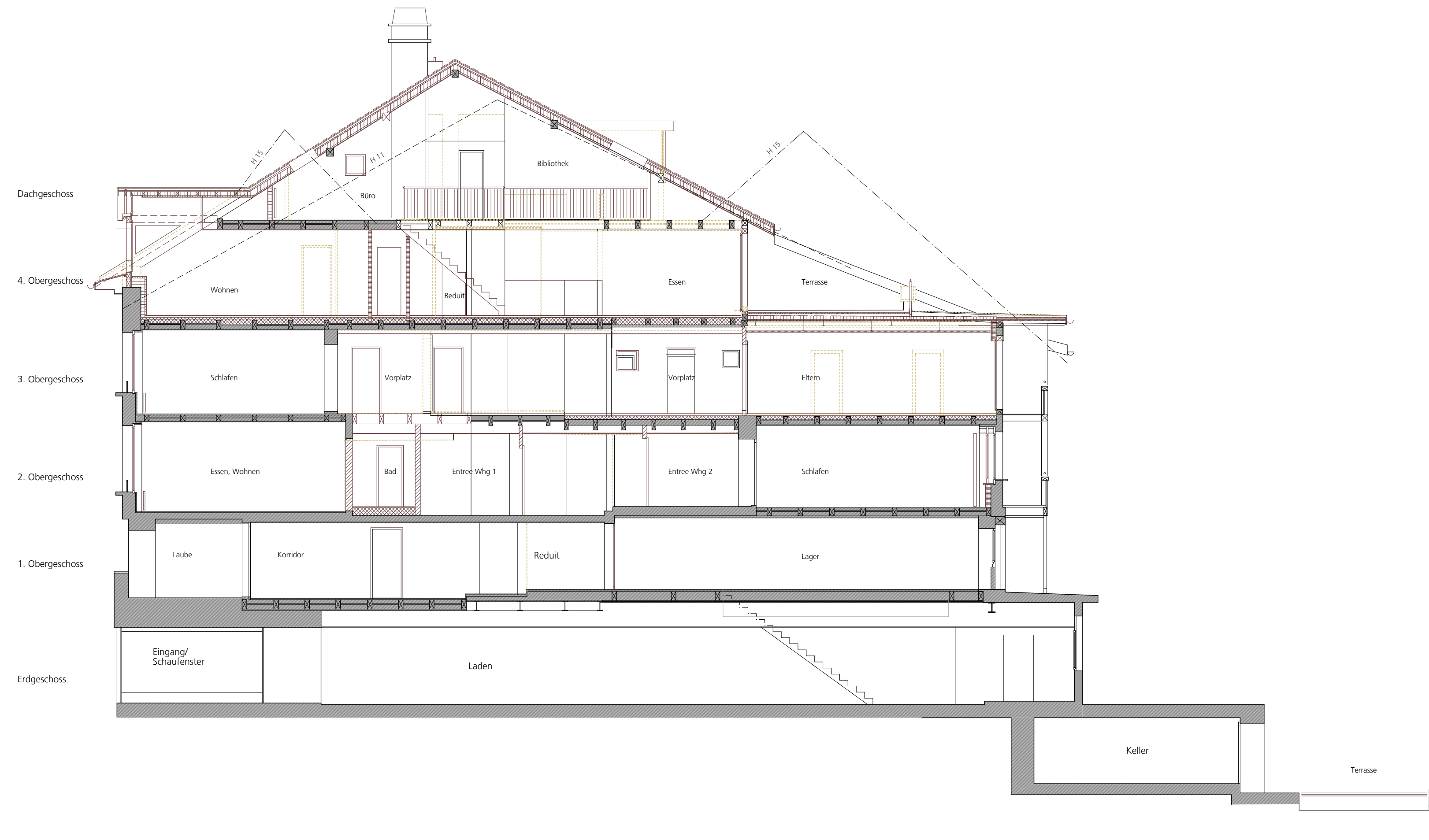
Längsschnitt
