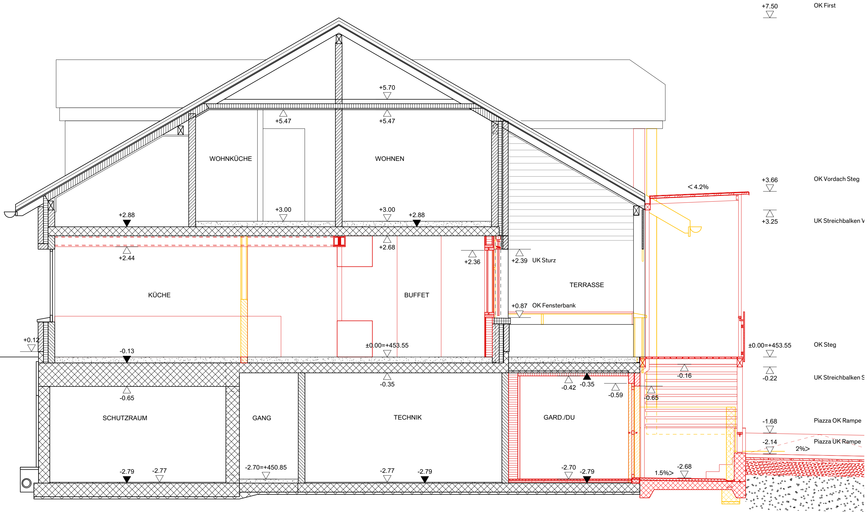
Schnitt GG
