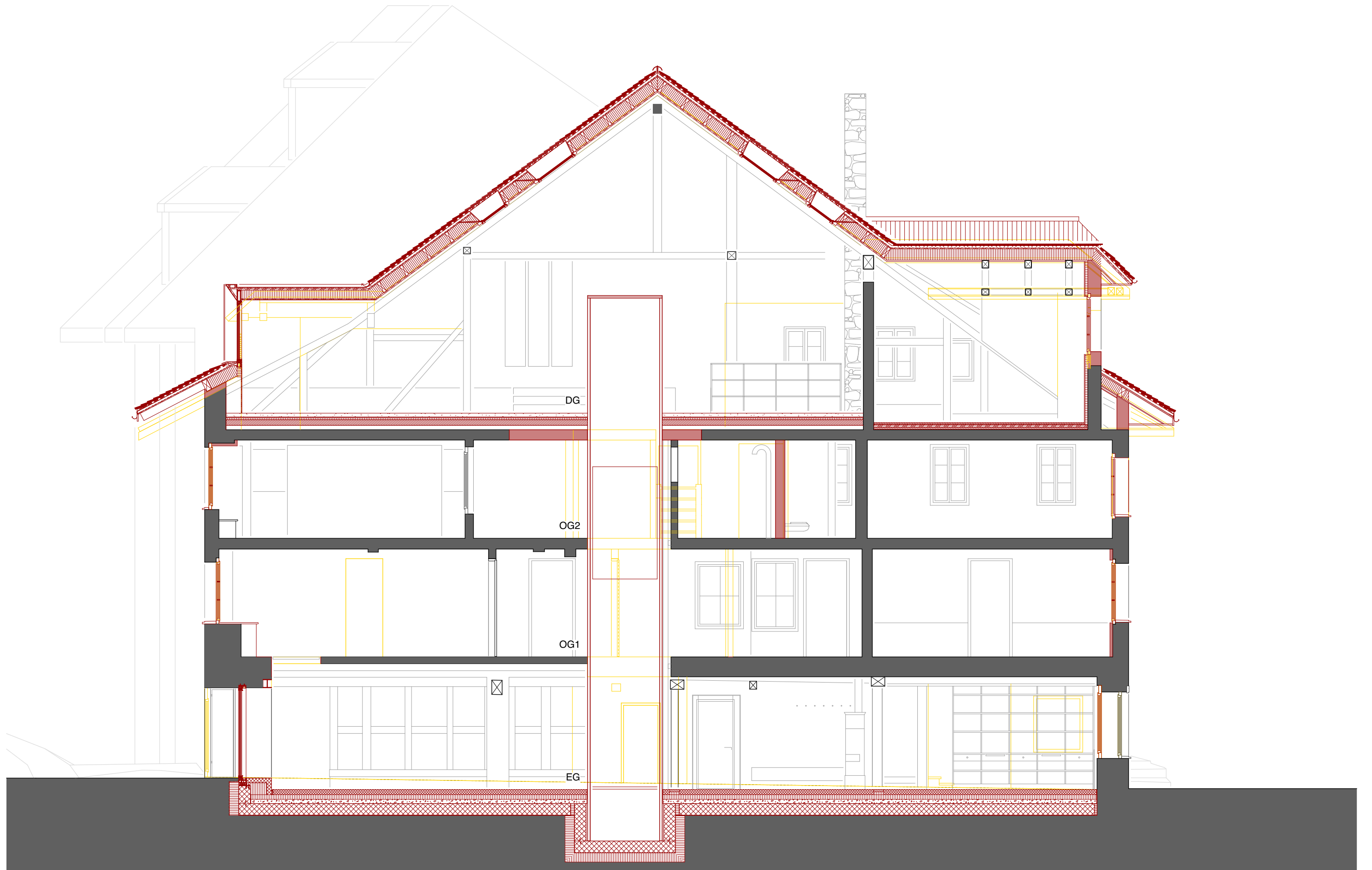
UMBAU WOHNHAUS HERRENRAIN 14 ALTSTADT SURSEE LÄNGSSCHNITT AMBERG ARCHITEKTEN AG SURSEE
