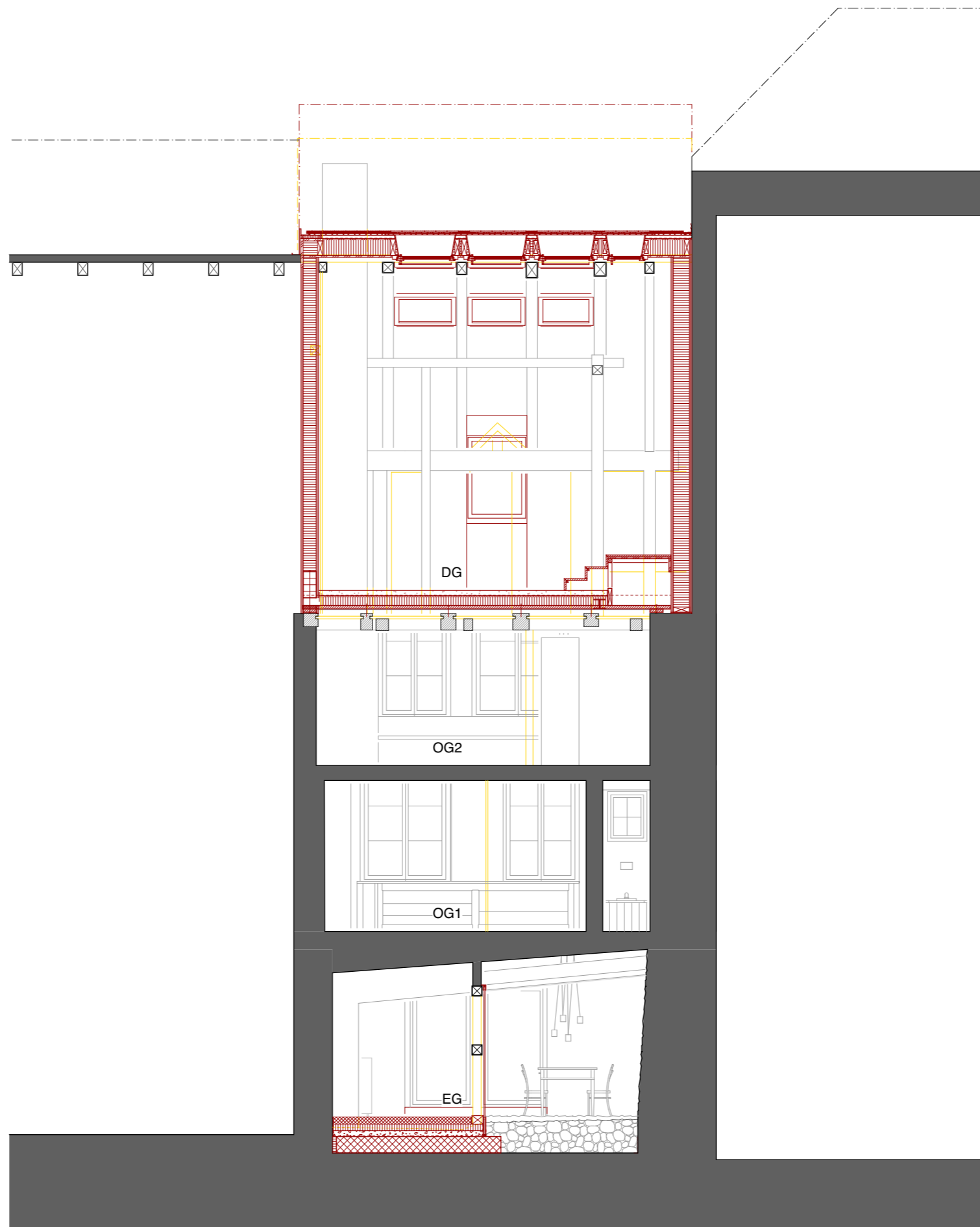
UMBAU WOHNHAUS HERRENRAIN 14 ALTSTADT SURSEE QUERSCHNITT AMBERG ARCHITEKTEN AG SURSEE
