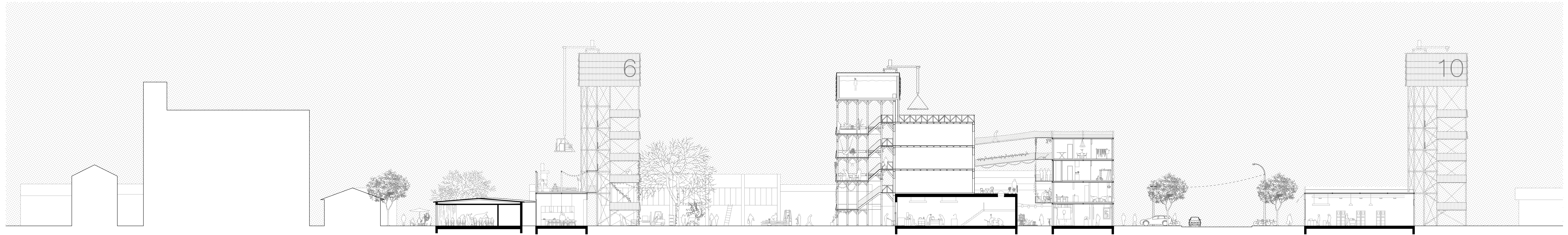
Längsschnitt 1:200
