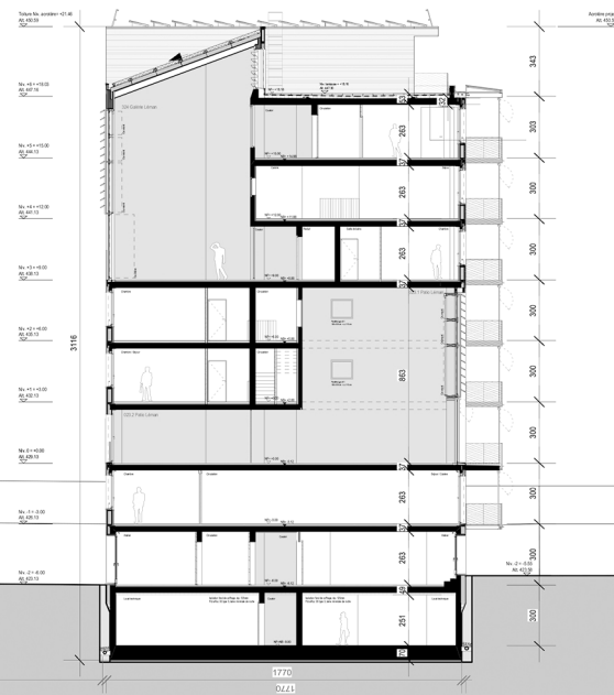
A11_Coupe AA
