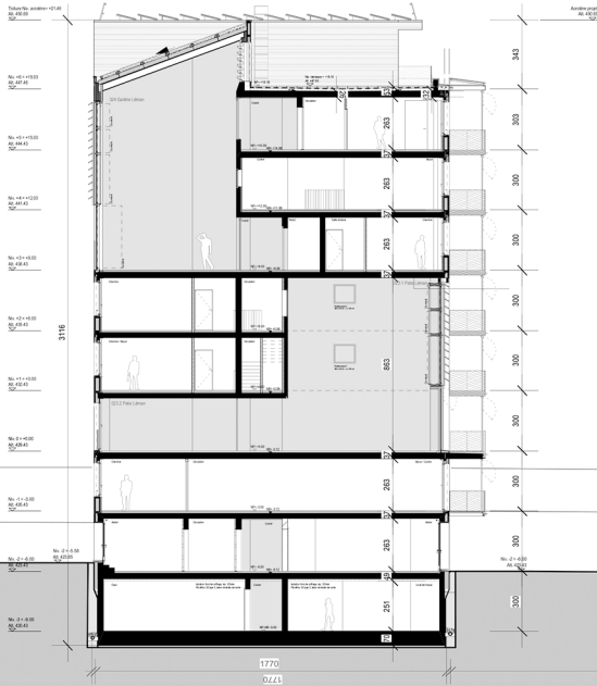
A12 Coupe AA
