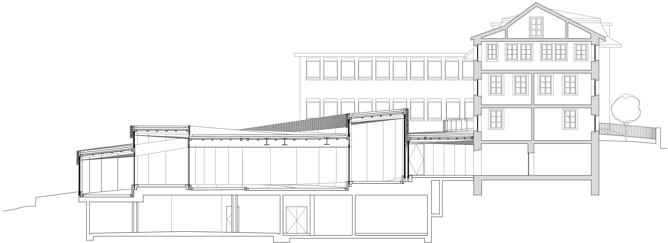
Coupe transversale - 1:200
