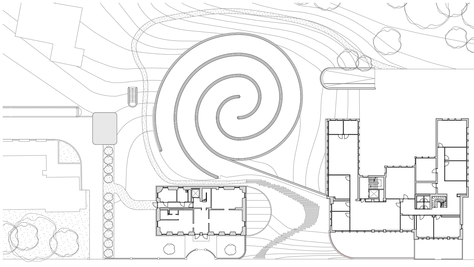
Toiture - 1:500
