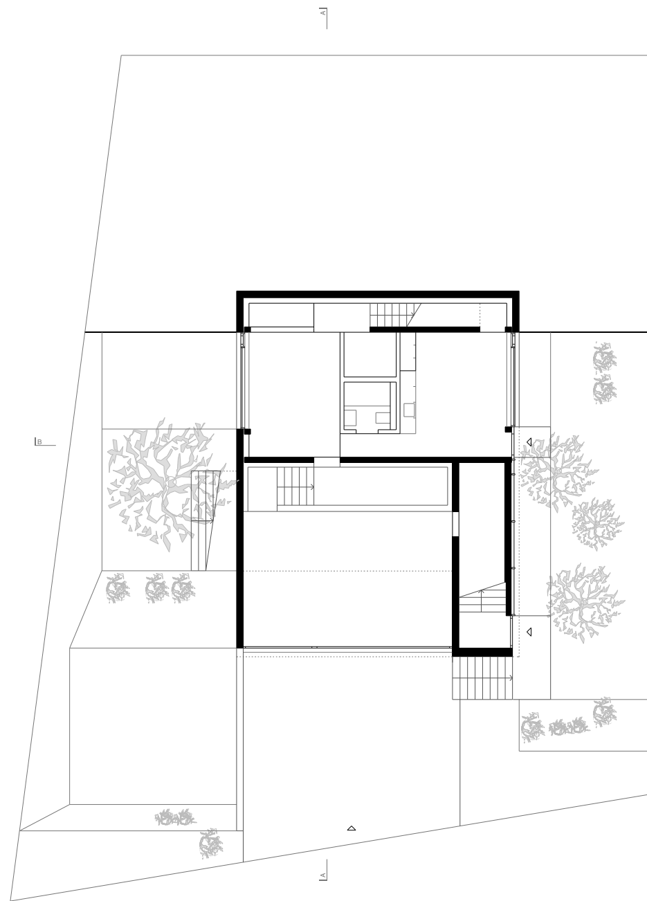
Haus Baumann - Grundriss Untergeschoss
