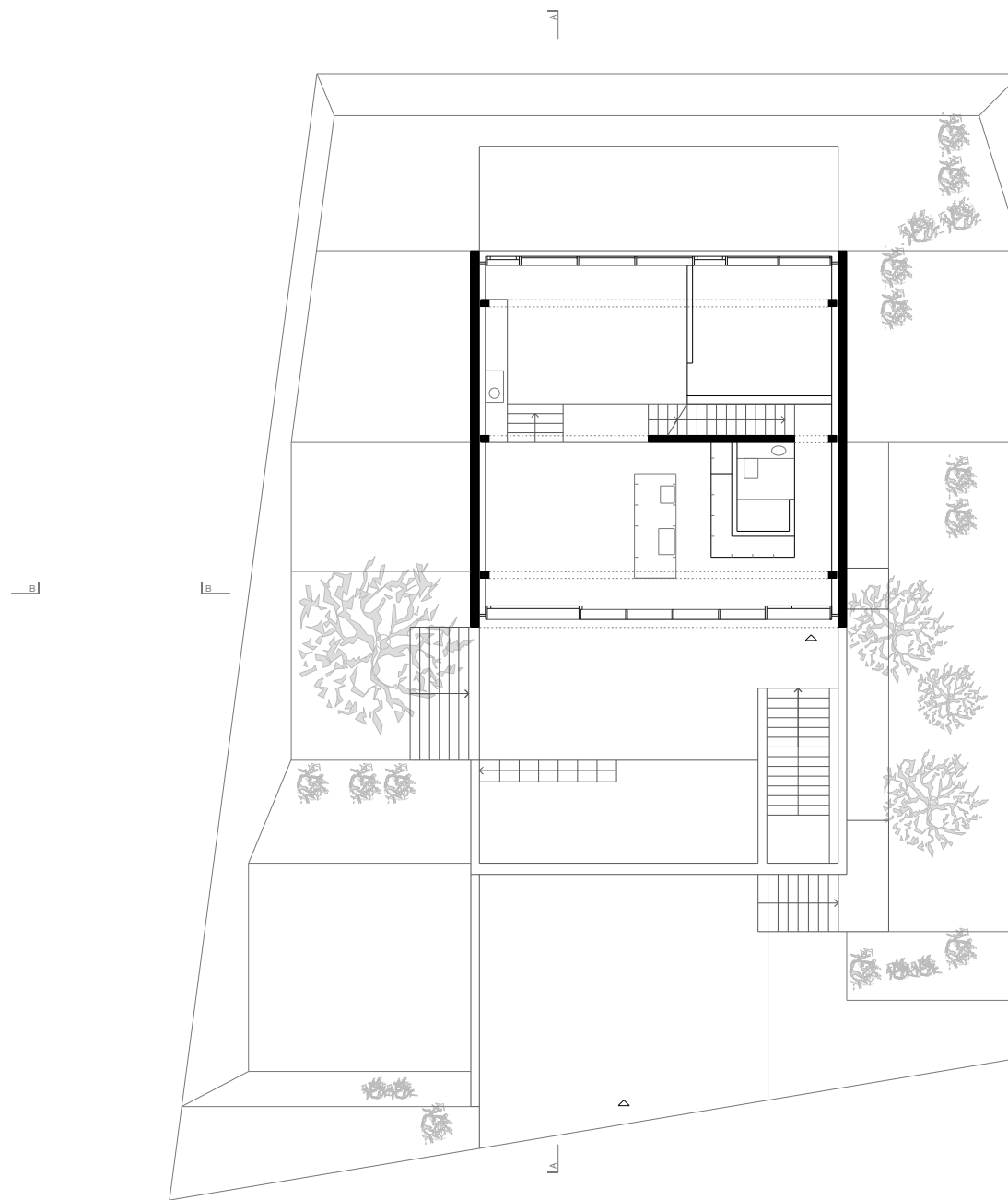
Haus Baumann - Grundriss Erdgeschoss
