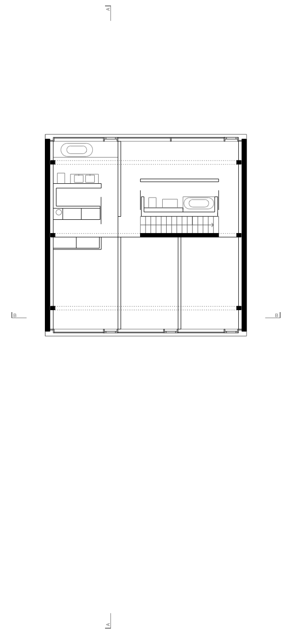
Haus Baumann - Grundriss Obergeschoss
