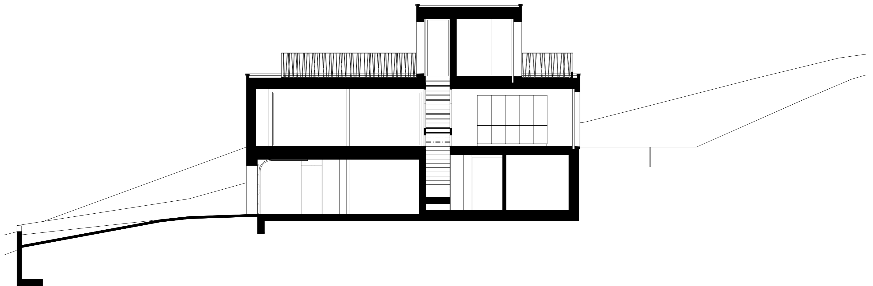
Schnitt B
