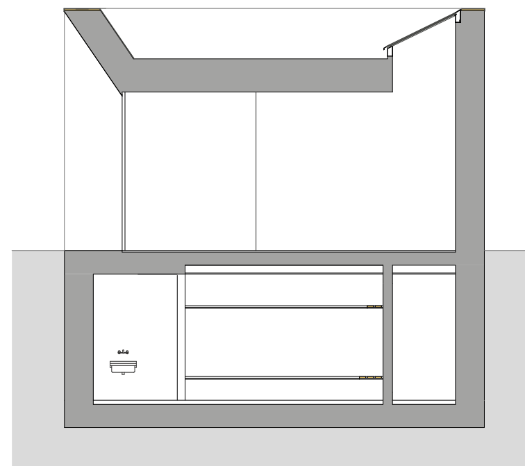
Schnitt C
