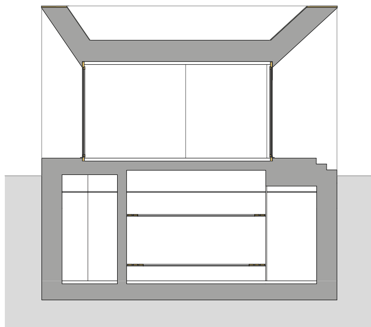
Schnitt B
