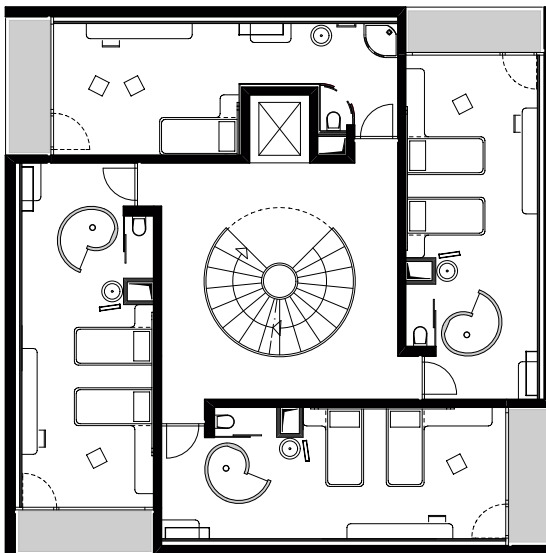
Pianta terzo piano
