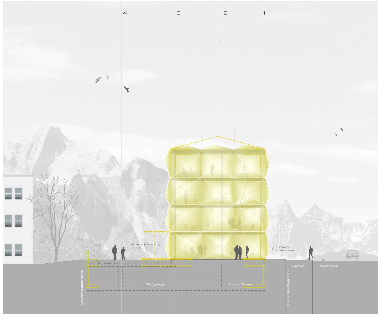
ANSICHT NORD
