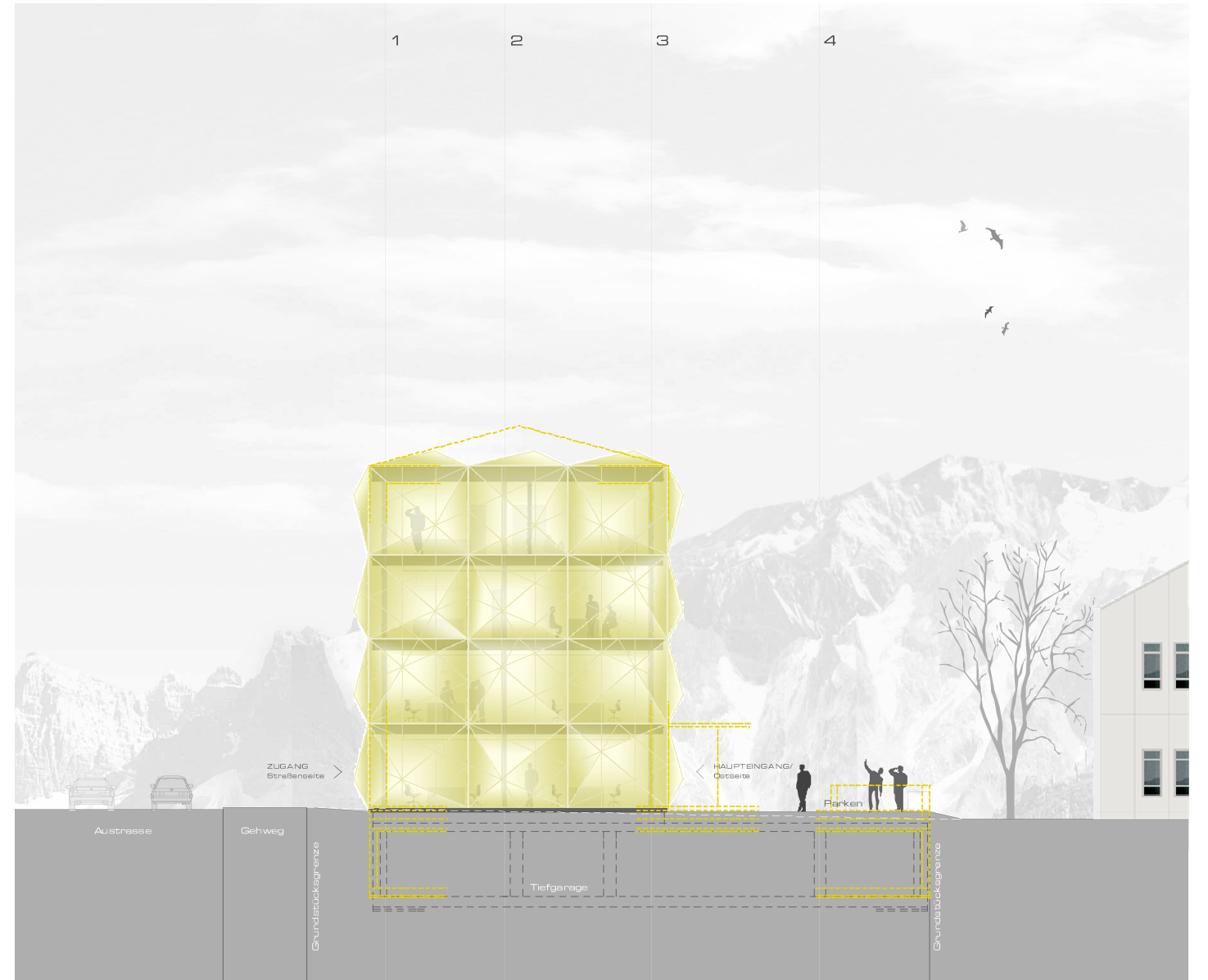
ANSICHT SÜD
